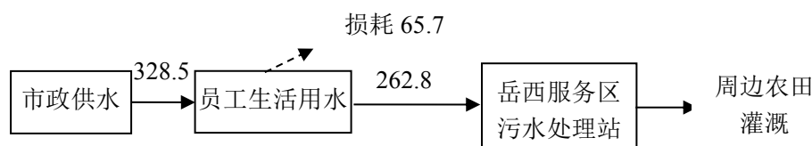
图 2.7 项目水平衡图 (m³/a)
