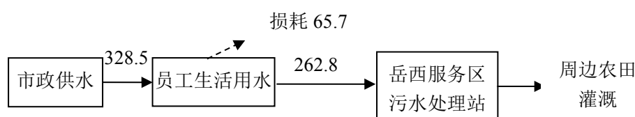
图 2.7 项目水平衡图 (m³/d)
