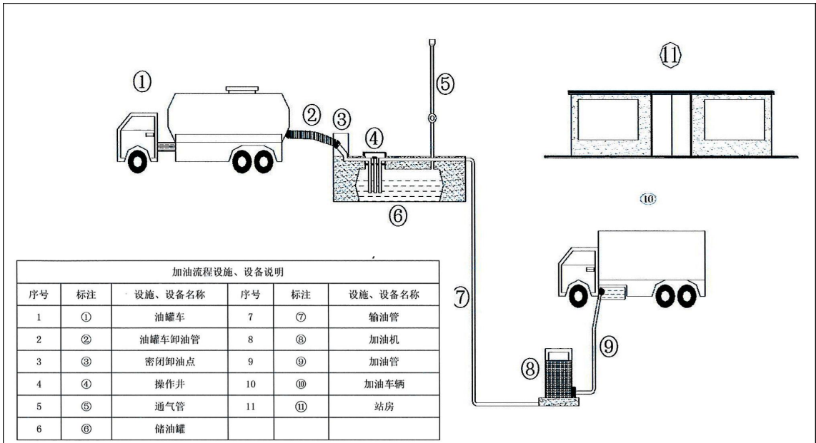
图 2.8-1 加油站工艺流程图
