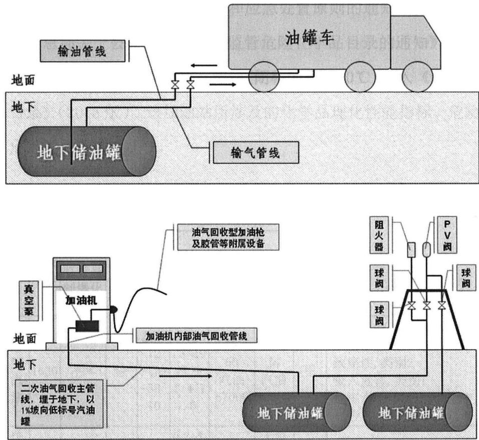
图 2.8-2 油气回收系统示意图
