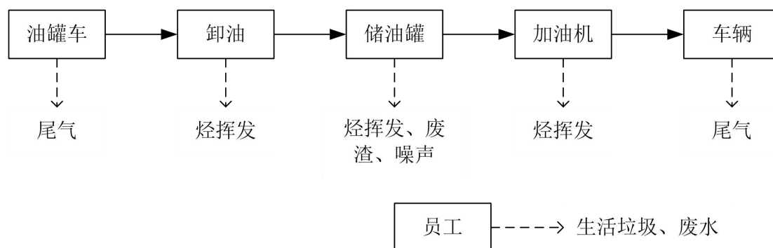
图 2.8-3 运营期工艺流程及产物环节示意图
