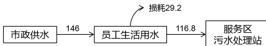
图 2.7 项目水平衡图 (m 3 /a)
