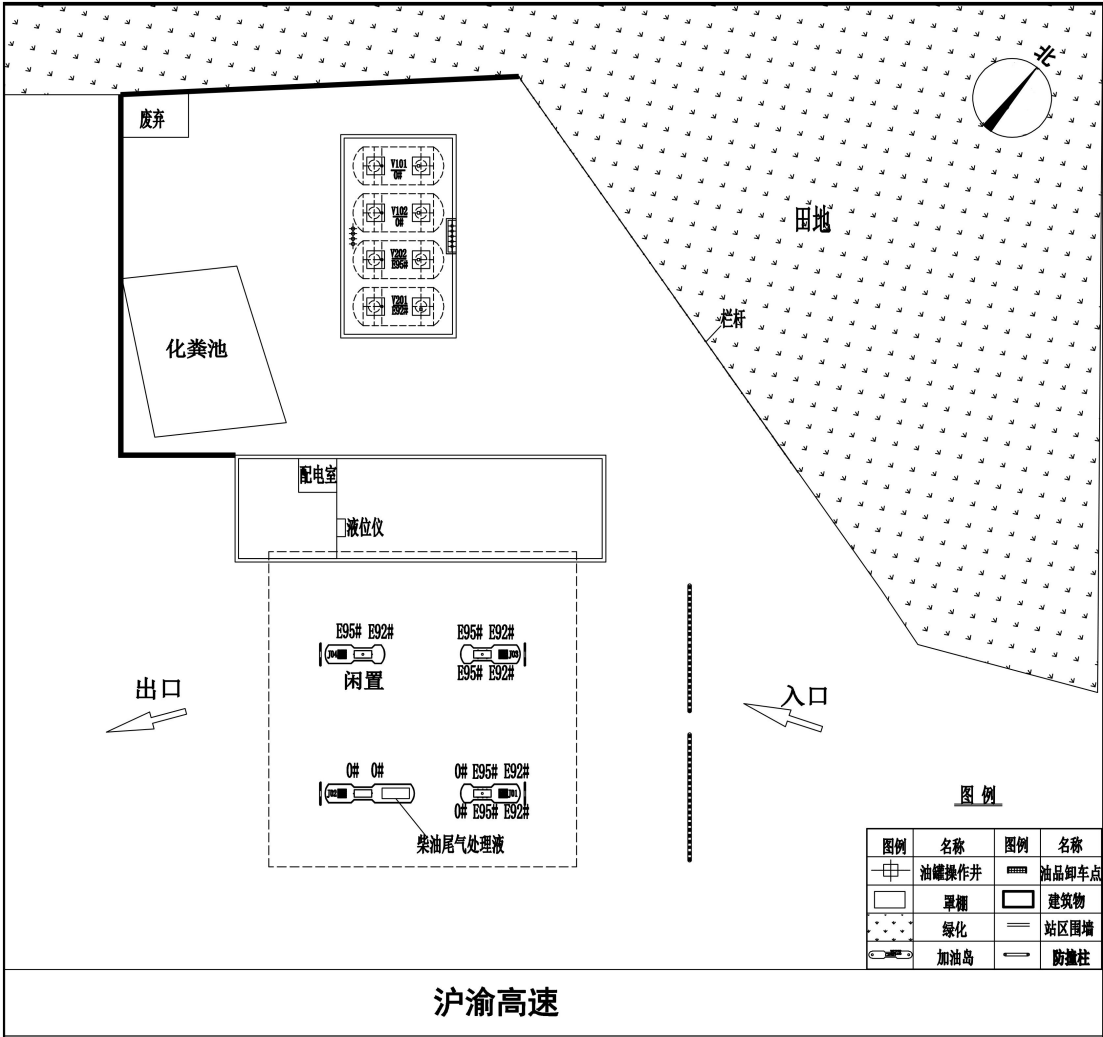
附图 2：项目平面布置
