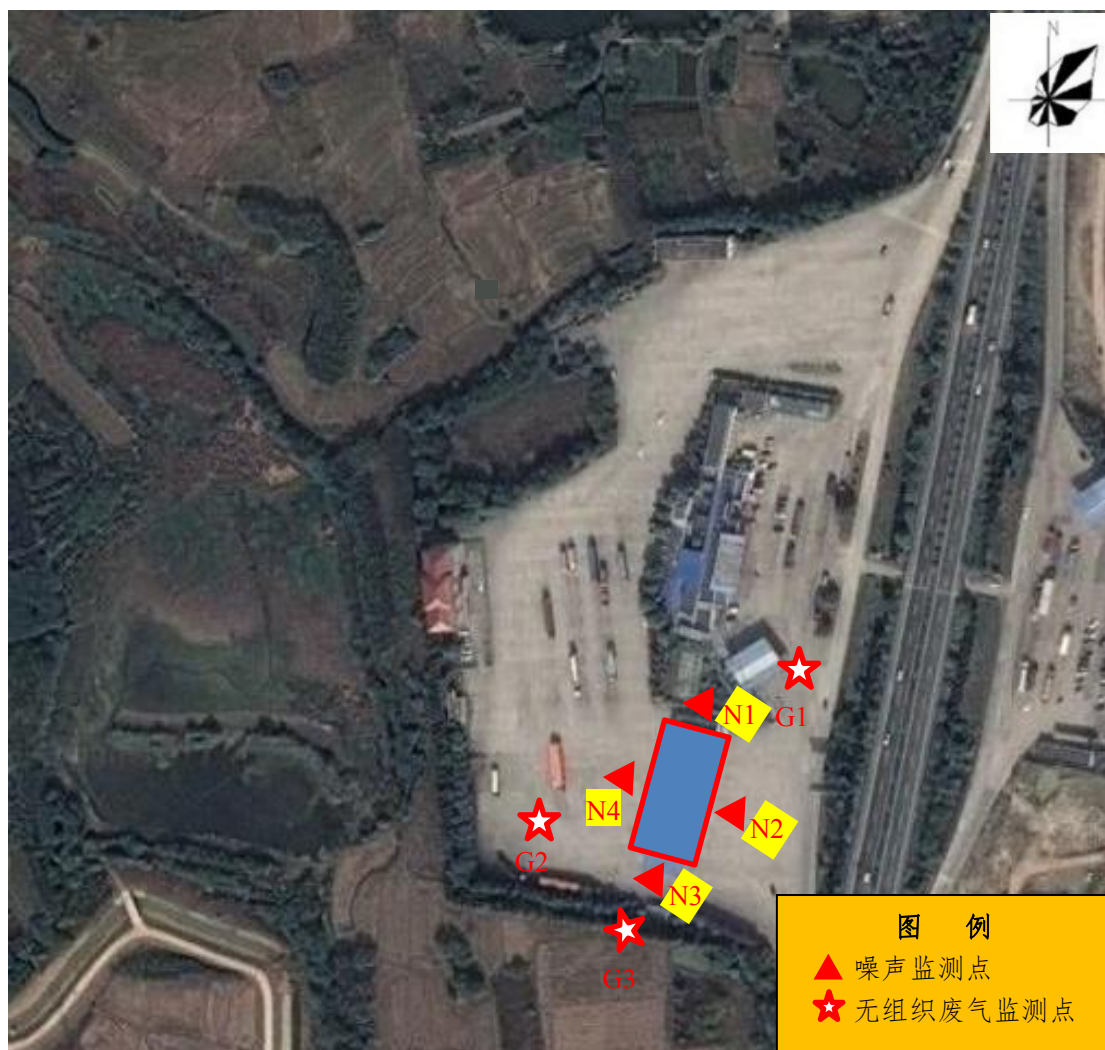
图 6-1 噪声及无组织废气监测点位图
