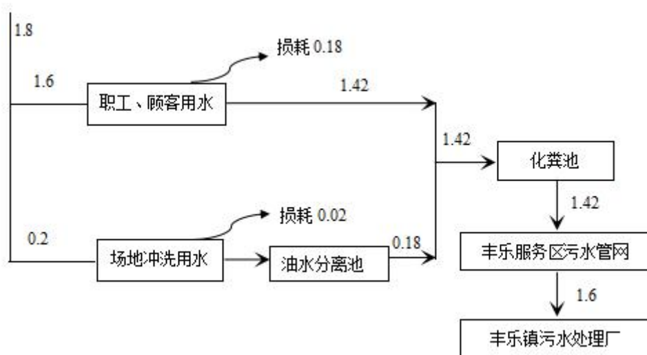
图 2.7 项目水平衡图 (m³/d)
