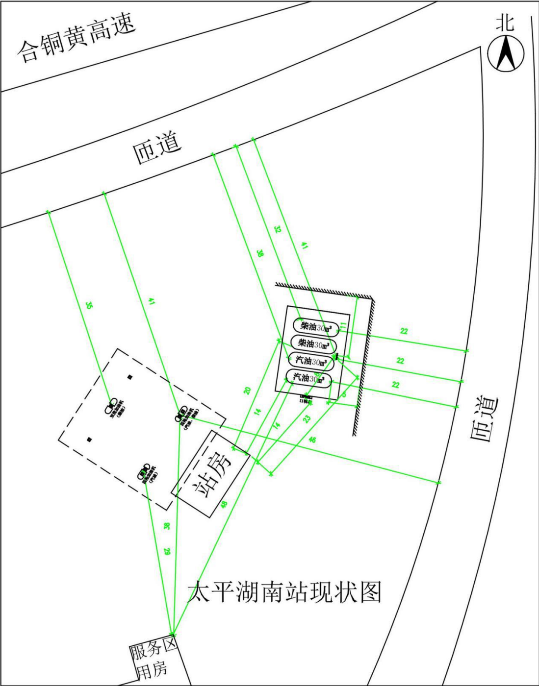
附图 2 加油站平面布置图
