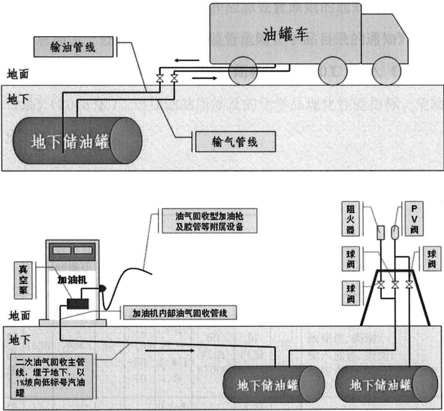
图 2-3 油气回收系统示意图
